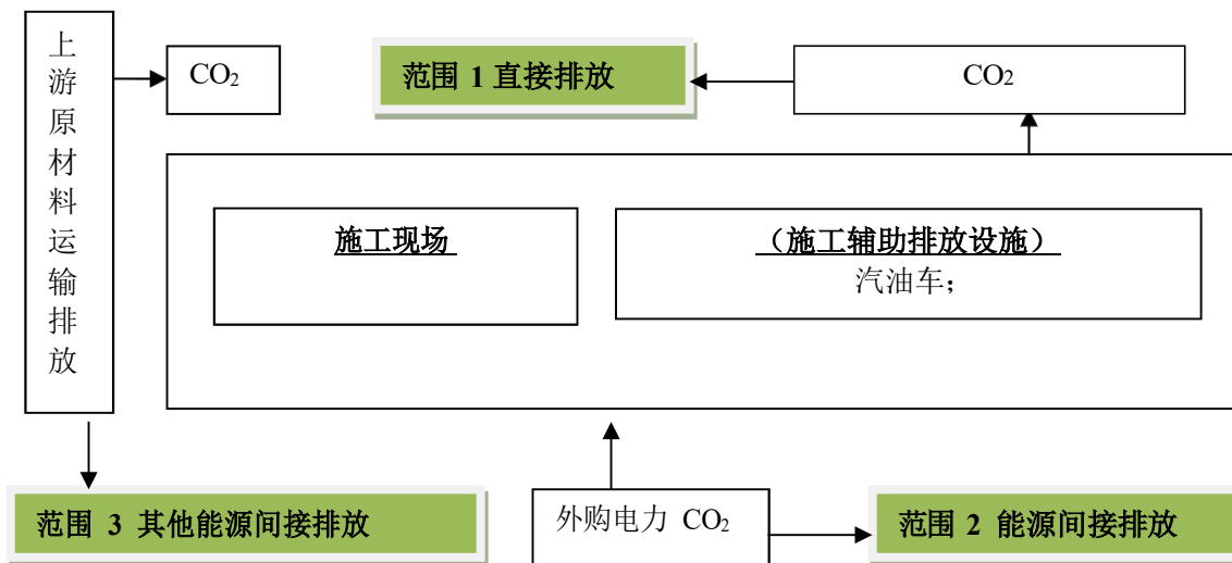
图 1 报告边界
